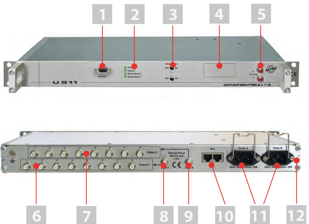
Bild 1: U 911 SAT-Verteilfeld
