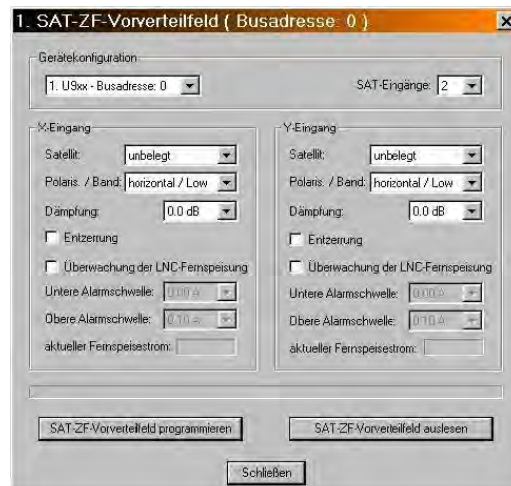
Bild 3: SAT-ZF-Vorverteilerfeld
